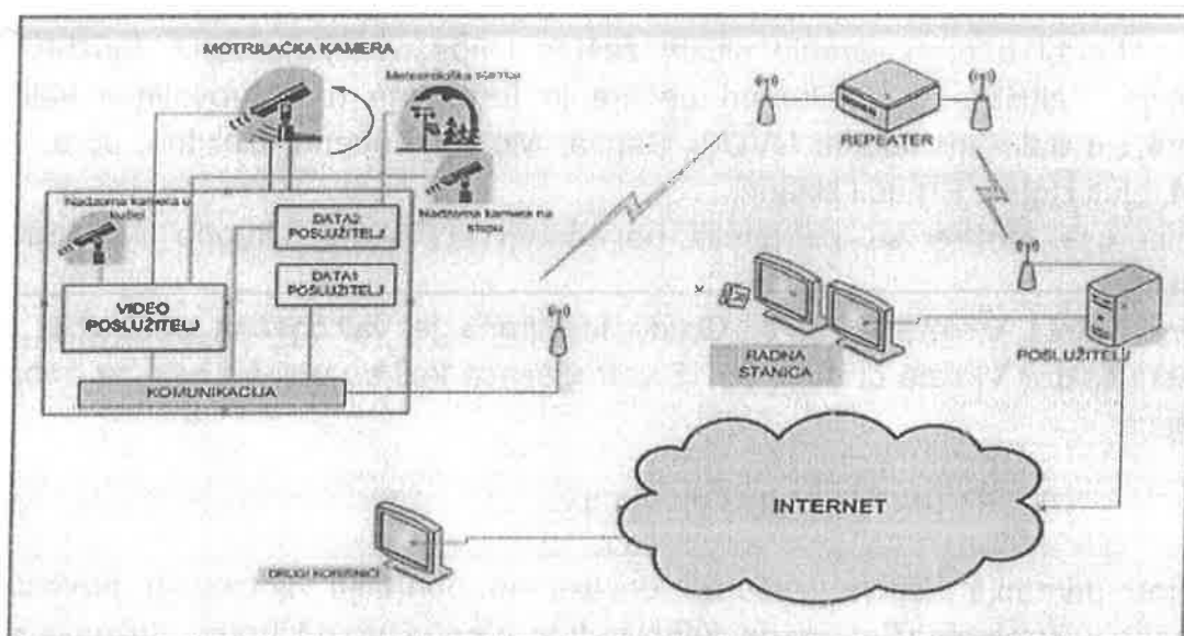
Slika 1. Osnovna blok shema cjelokupnog sustava
