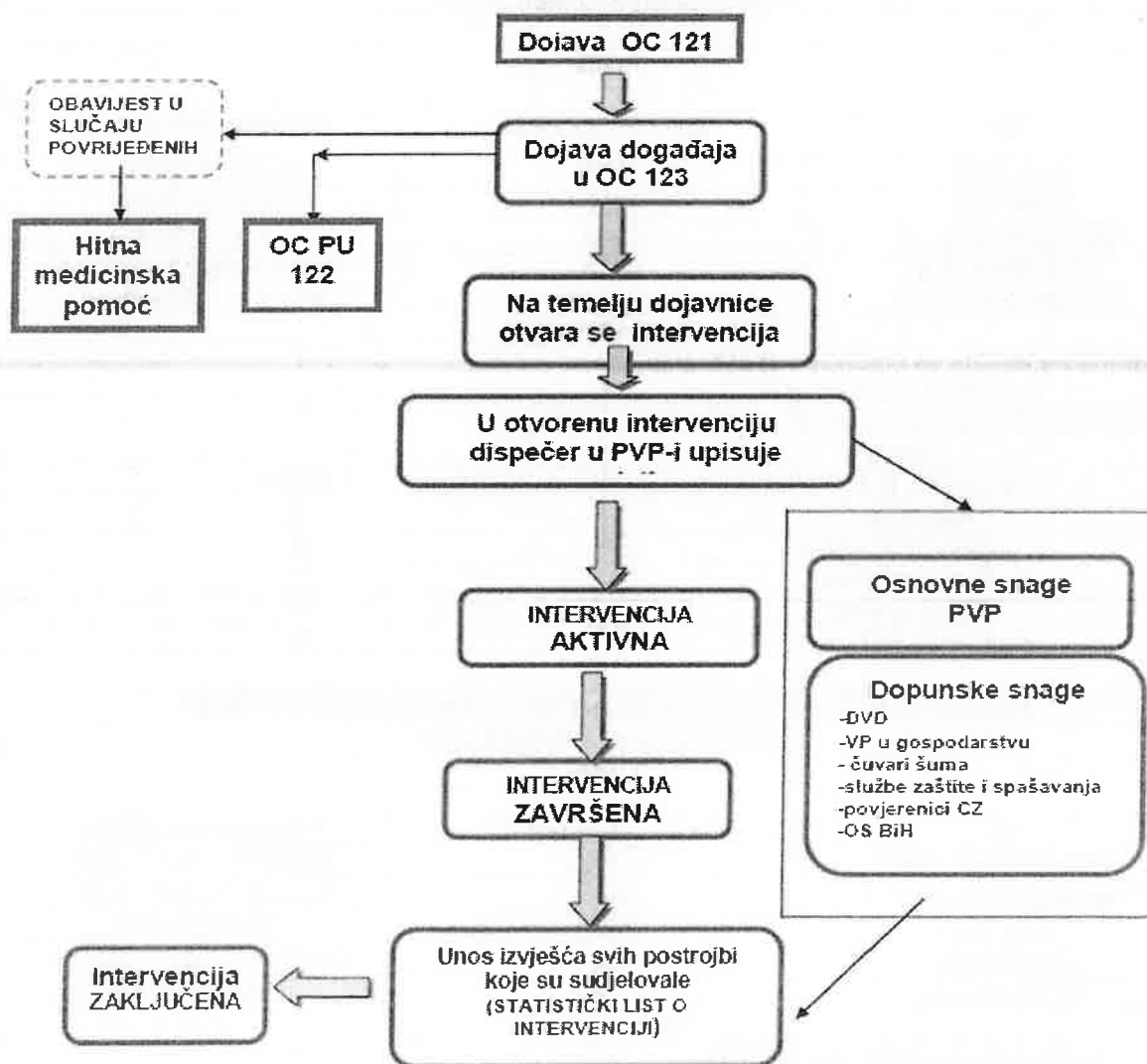
Slika 2. Shema uzbunjivanja u slučaju požara većih razmjera
