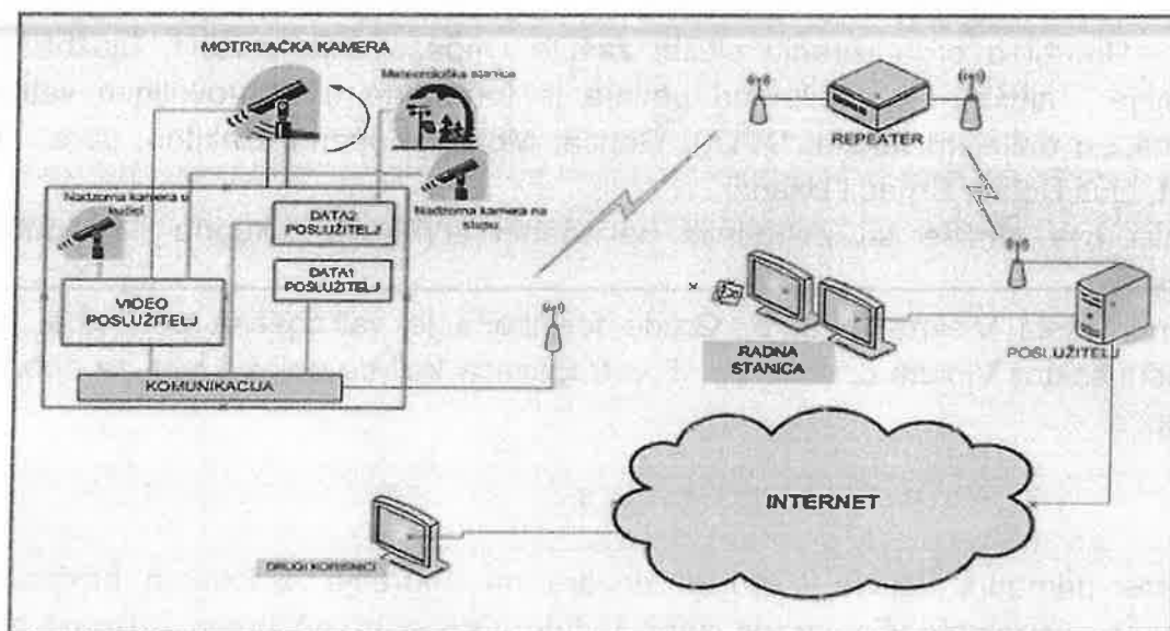
Slika 1. Osnovna blok shema cjelokupnog sustava
